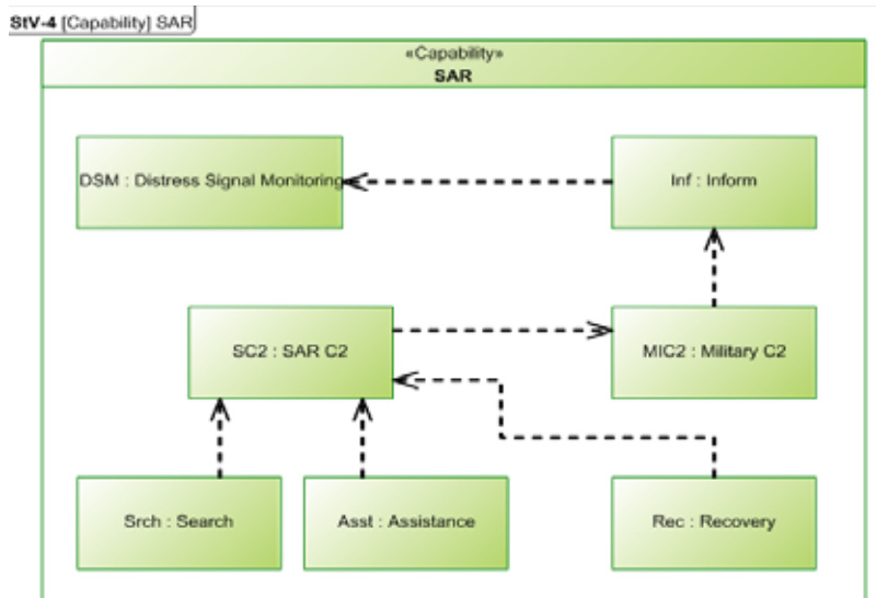
Figure D.9 - StV-4
