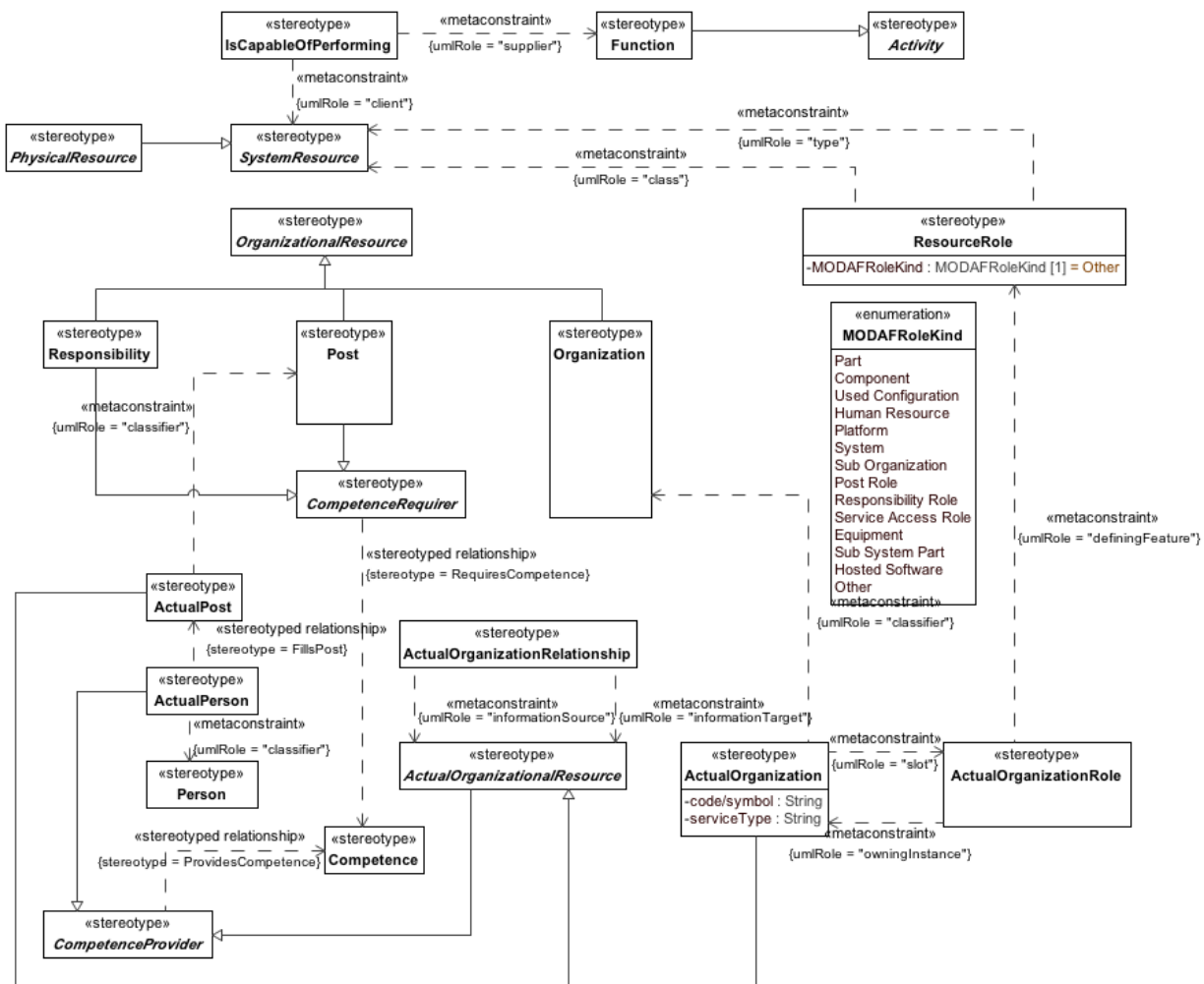
Figure B.12 - OV-4 Actual
