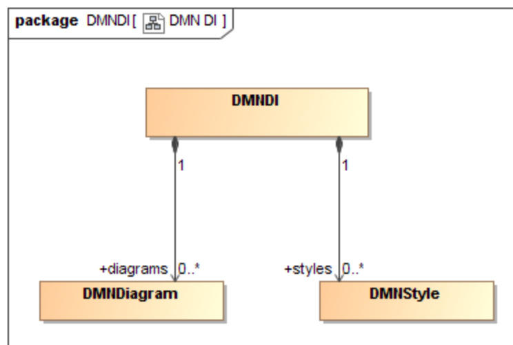
Figure 13-1: DMNDI
