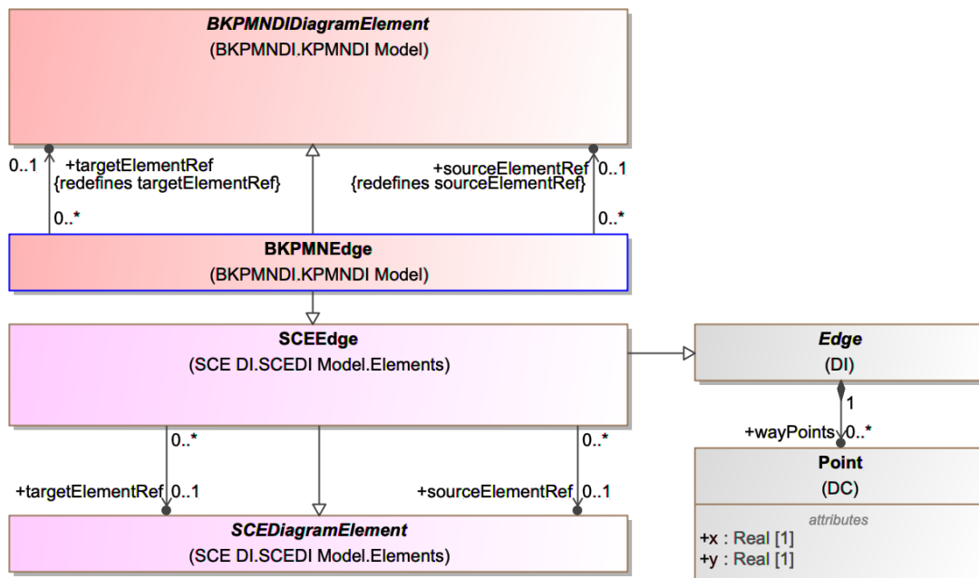
Figure 78: BKPMNDI Edge
